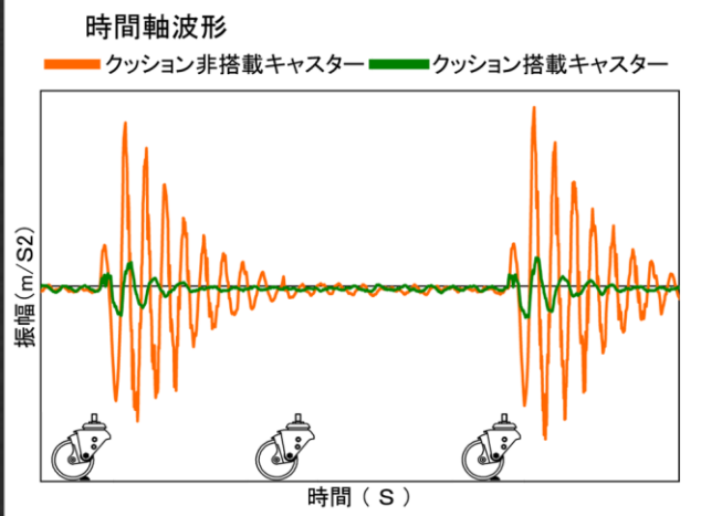
従来品キャスターとクッション搭載キャスターの振動加速度比較
